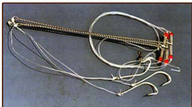
ML-09 Pateranoster 10 cm. Arm
